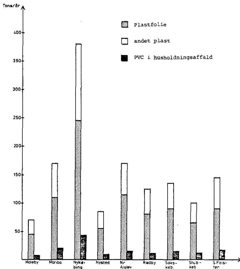
Fig. 2.4 Illustration af plastmængder og kvaliteter i dagrenovation
