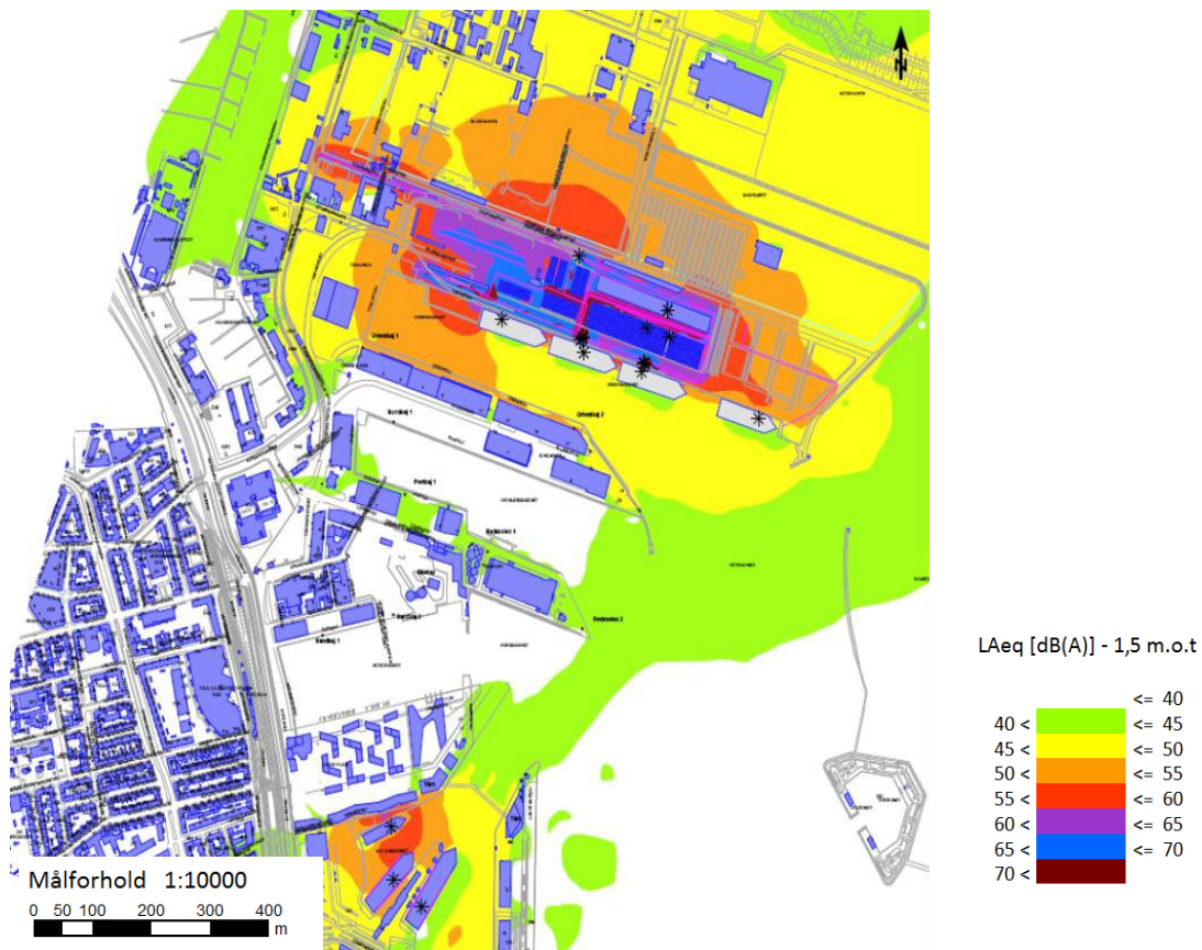
Figur 7.18: Støj kort fra en tidligere undersøgelse, som viser støjdbredelsen fra den eksisterende container-terminal, og færgeterminal i mellembassinet. kilde: Miljørapport for udflytning af containerterminalen til Ydre Nordhavn, Grontmij oktober 2011. Støj kortet er udarbejdet af COWI i forbindelse med udvikling af Århusgade området, d. 29.11.2010.
