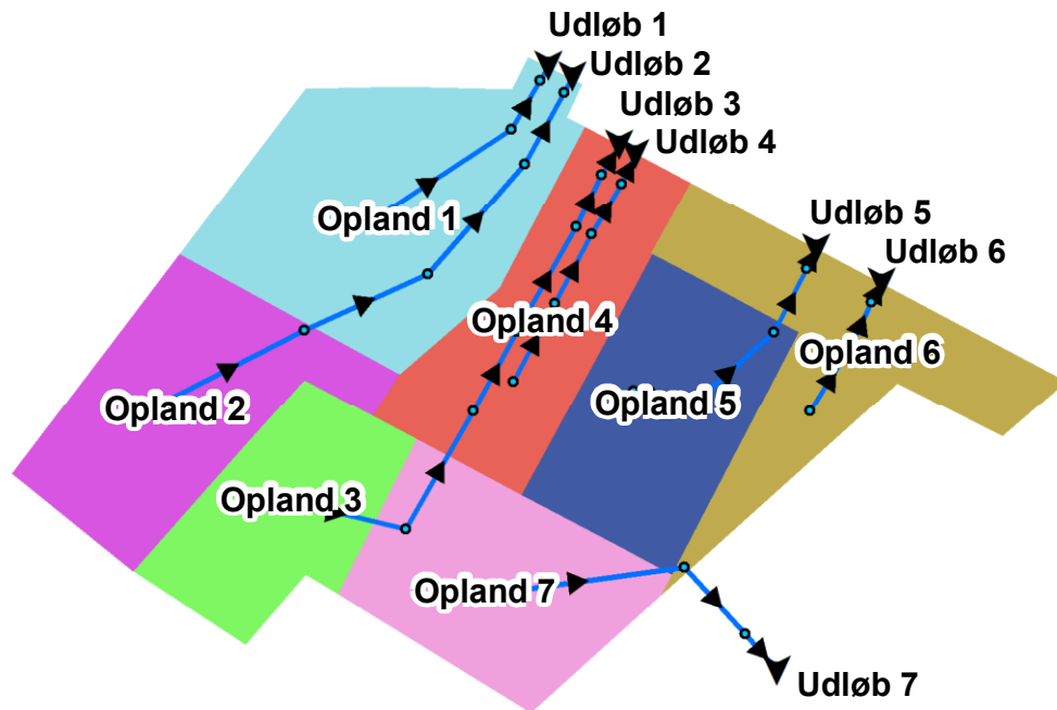
Figur 2.5 Skitse af planlagt afvandingssystem (blå linjer) med deloplande 4, 5 og 6 for containerterminal, 1 og 2 for ro-ro anløbsplads samt 3 og 7 for fællesareal.
