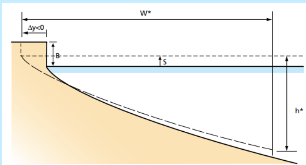
Figur 11-3. Bruuns Regel. Skitse af kystrespons pga. vandstandsstigning. Tilbagerykningen findes som \Delta y = \frac{S}{W} (W^* I (h^* + B))^{180} .
