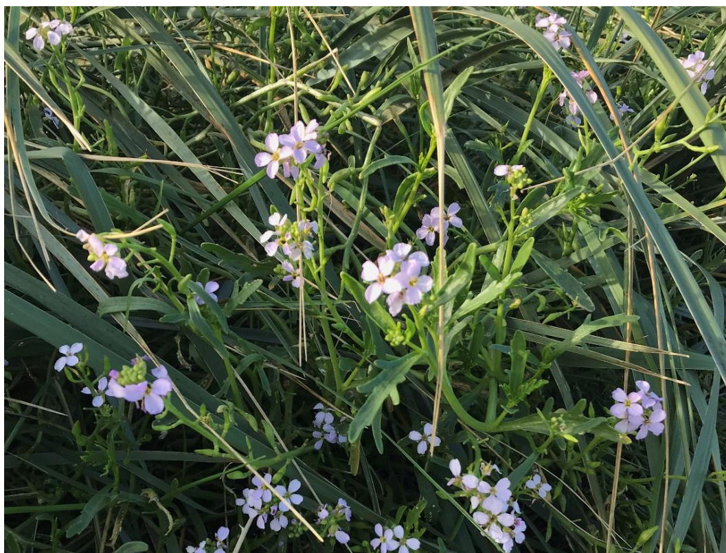
Figur 16-7. Strandsennep i den grønne klit langs strækningen ved Blåvand.
