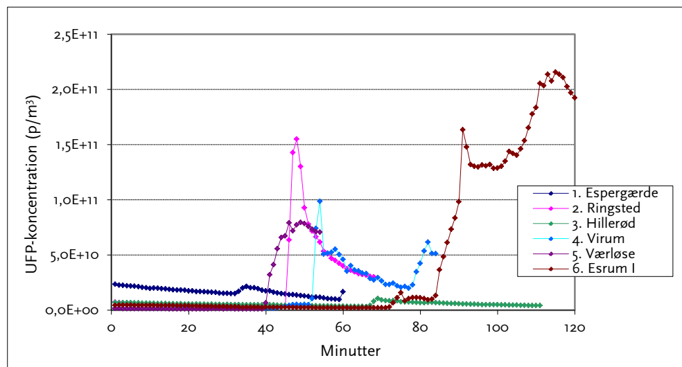
FIGUR 11. FIGUREN VISER UDVIKLINGSFORLØBET FOR PARTIKELMISSIONEN FRA DE RESPEKTIVE OVNE MÅLT I 2. MÅLESERIE. DE STOR PARTIKELUDSLIP OPSTÅR TYPISK VED OPTÆNDING OG PÅFYLDNING AF OVNE, DVS. NÅR OVNLÅGEN HOLDES ÅBEN.
