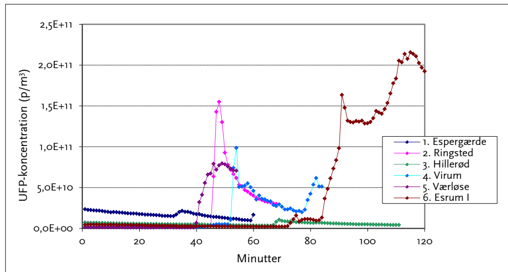
FIGUR 11. FIGUREN VISER UDVIKLINGSFORLØBET FOR PARTIKELEMISSIONEN FRA DE RESPEKTIVE OVNE MÅLT I 2. MÅLESERIE. DE STOR PARTIKELUDSLIP OPSTÅR TYPISK VED OPTÆNDING OG PÅFYLDNING AF OVNE, DVS. NÅR OVNLÅGEN HOLDES ÅBEN.
