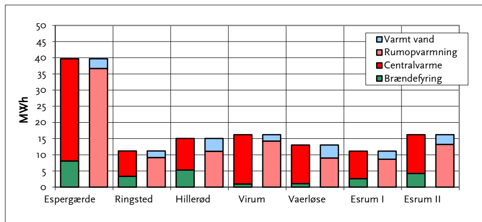
FIGUR 1. VARMEBALANCER, SOM FOR DET ENKELTE HUS ILLUSTRERER OMFANGET AF DEN VARME-PRODUKTION, DER FINDER STED - HER BRÆNDEFYRING OG CENTRALVARME - OVER FOR STØRRELSEN AF DET BEREKNEDNE FORBRUG, DVS. BIDRAGET TIL RUMOPVARMNING OG VARMT BRUGSVAND, JF. FIGUR 5 I RAPPORTEN.
