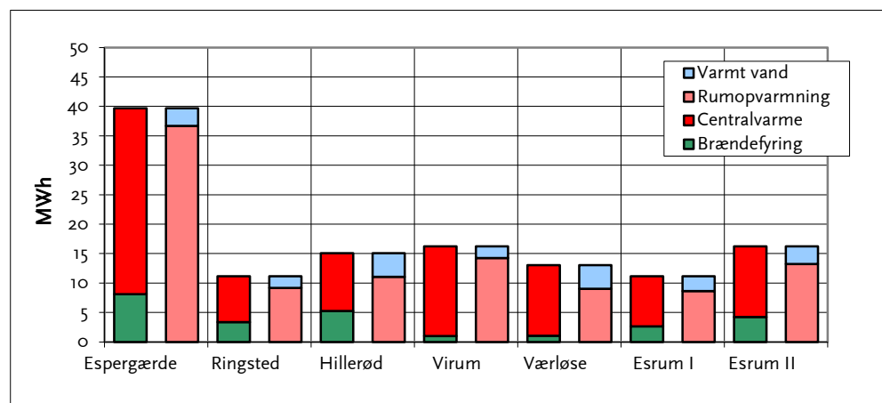
FIGUR 5. VARMETILFØRSELN, SOM FOR DET ENKELTE HUS ILLUSTRERER OMFANGET AF DEN VARMETILFØRSEL, DER FINDER STED, HER BRÆNDEFYRING OG CENTRALVARME, STILLET OP OVER FOR DET FORBRUG, DER ER ESTIMERET, HER FORDELT PÅ RUMOPVARMNING OG VARMT BRUGSVAND
