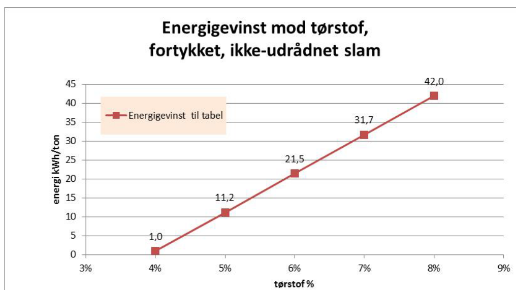
Figur 1 Energigevinst af fortykket, ikke-udrådnet slam.
