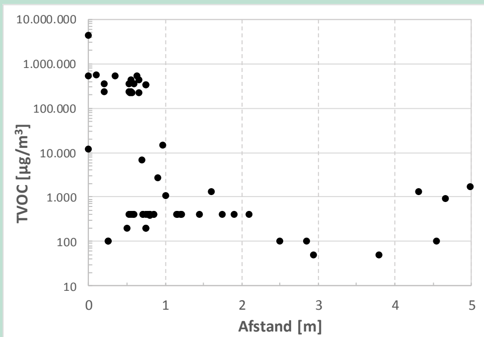
FIGUR 8. Samlet datasæt for TVOC-koncentration i poreluft som funktion af afstanden til kilden/jordforurening indenfor 5 meter til kilde/jordforurening (logaritmisk koncentrationsakse).
