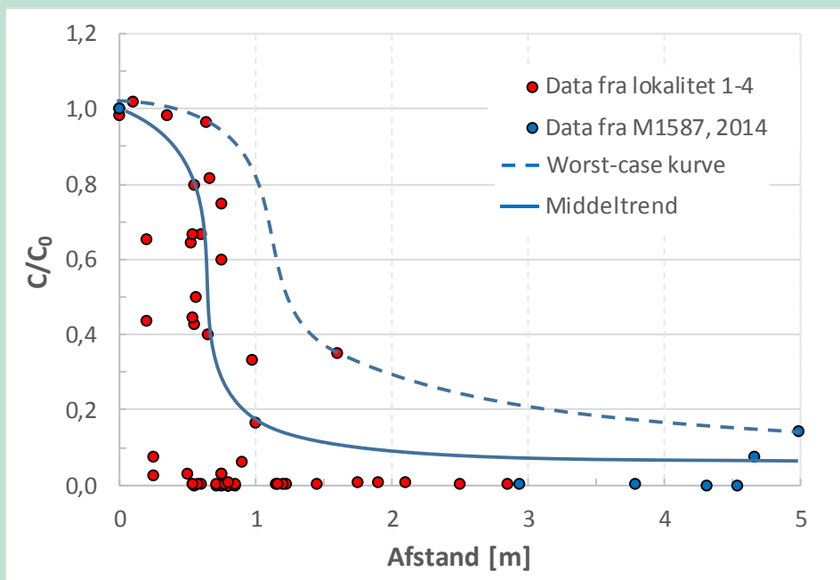
FIGUR 5. Relativ TVOC-koncentration ( C/C_0 ) som funktion af afstand til kil- den/jordforureningen (maks. afstand 5 meter). I grafen er der indlagt eye-fittede kurver for worst-case trend og middeltrend.
