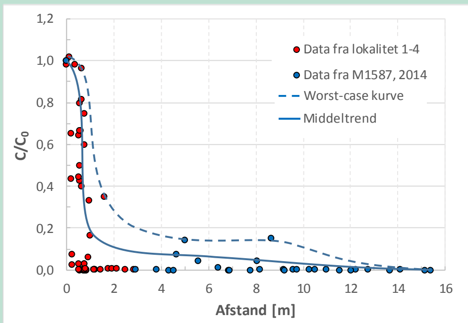
FIGUR 4. Relativ TVOC-koncentration ( C/C_0 ) som funktion af afstand til kil- den/jordforureningen (maks. afstand 16 meter). I grafen er der indlagt eye-fittede kurver for worst-case trend og middeltrend.
