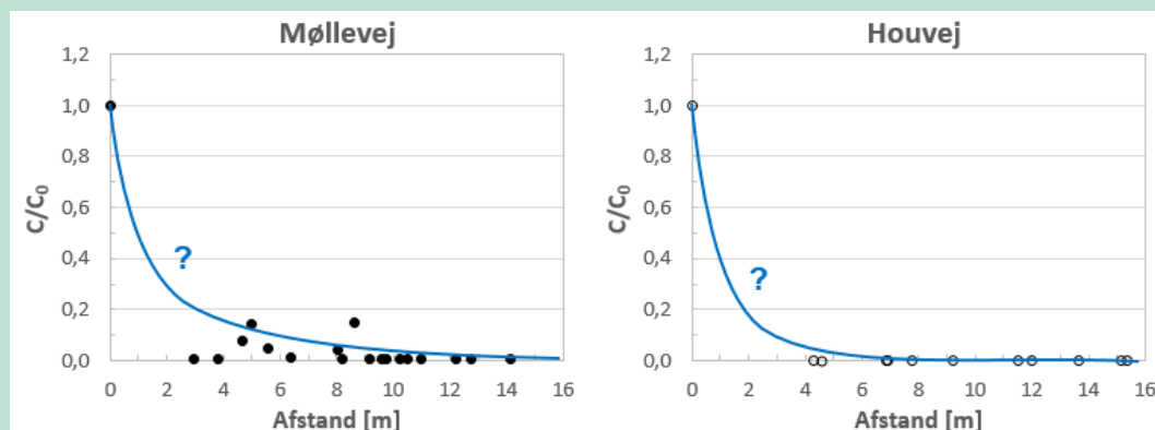
FIGUR 1. Relativ koncentration af oliekomponenter (TVOC) som funktion af afstanden fra kilden/jordforureningen, data fra /2/.
