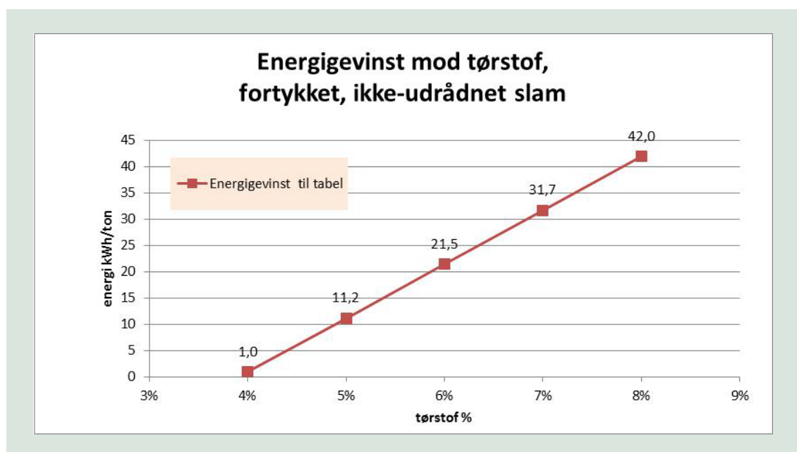
FIGUR 1. Energigevinst af fortykket, ikke-udrødnet slam
