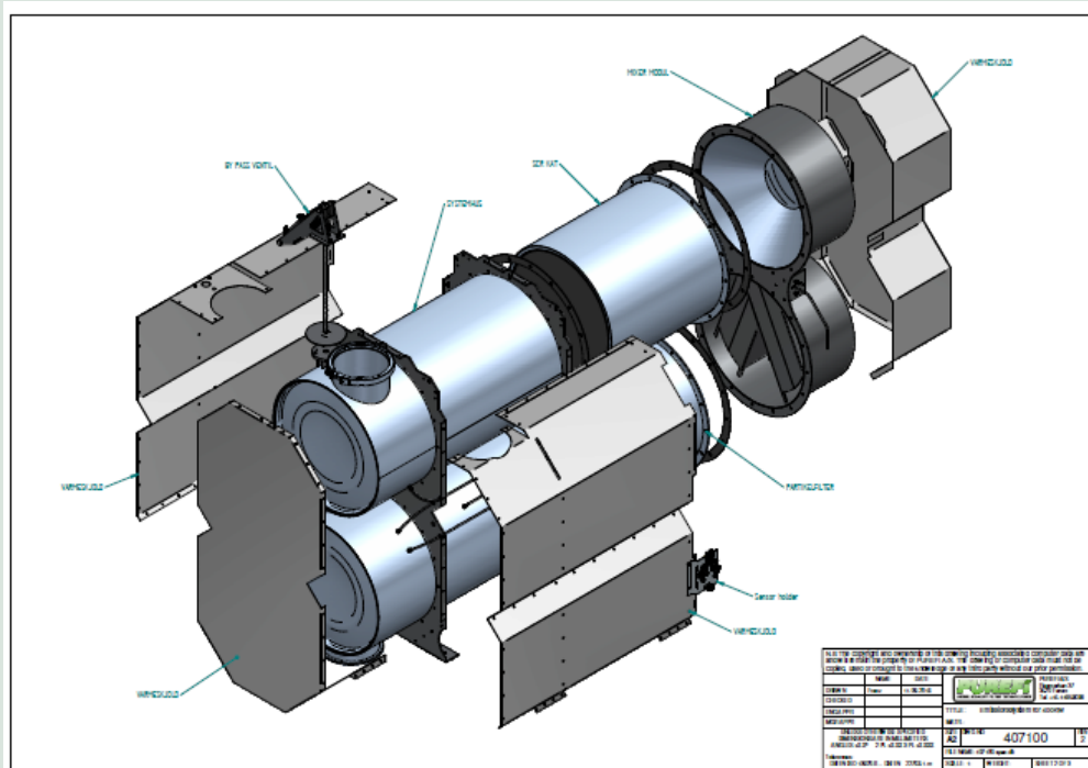
FIGUR 3. Enkelt emissionssystem med udvendig isolerende beklædning.
