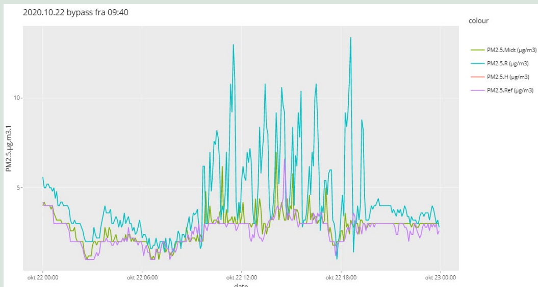
FIGUR 20. Data fra den 22. oktober 2020, hvor færgeren startede med at sejle kl. 6:15. Partikelfiltrenes bypass blev åbnet kl. 9:40 og først aktiveret igen efter færgerens sidste sejltur var gennemført kl. 19:40.
