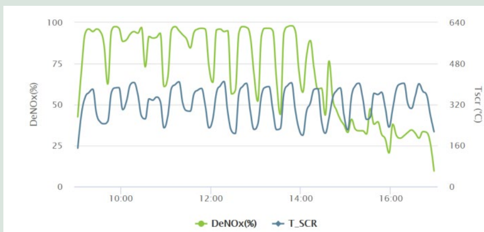
FIGUR 22. NO x reduktion med Amminex ASDS™ system.
