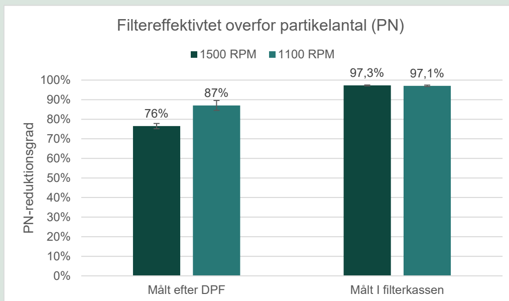
FIGUR 14. PN-reduktionsgrad i to forskellige målepunkter målt ved henholdsvis 1100 RPM og 1500 RPM.
