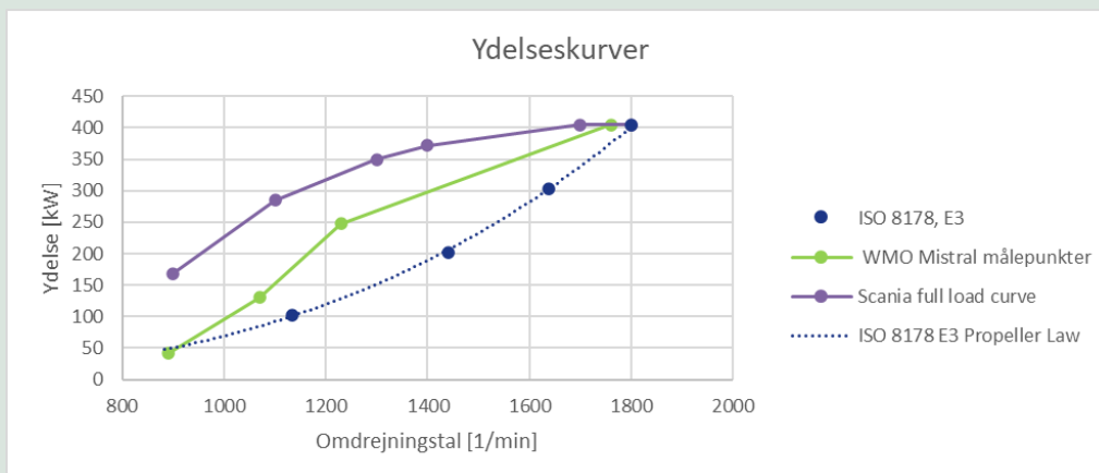
FIGUR 2. Grafen viser motorens effektkurve (øverst), målepunkter (midterst) og målepunkter på en idealiseret propeller-kurve jf. ISO 8178, E3 (nederst).
