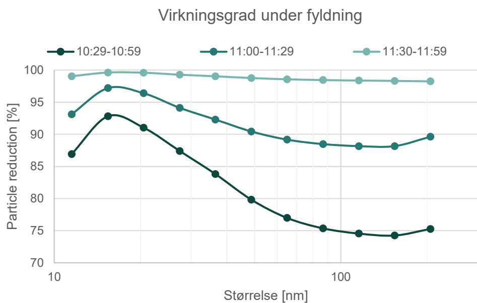
FIGUR 12. Visualisering af virkningsgrad som funktion af partikelstørrelse.
