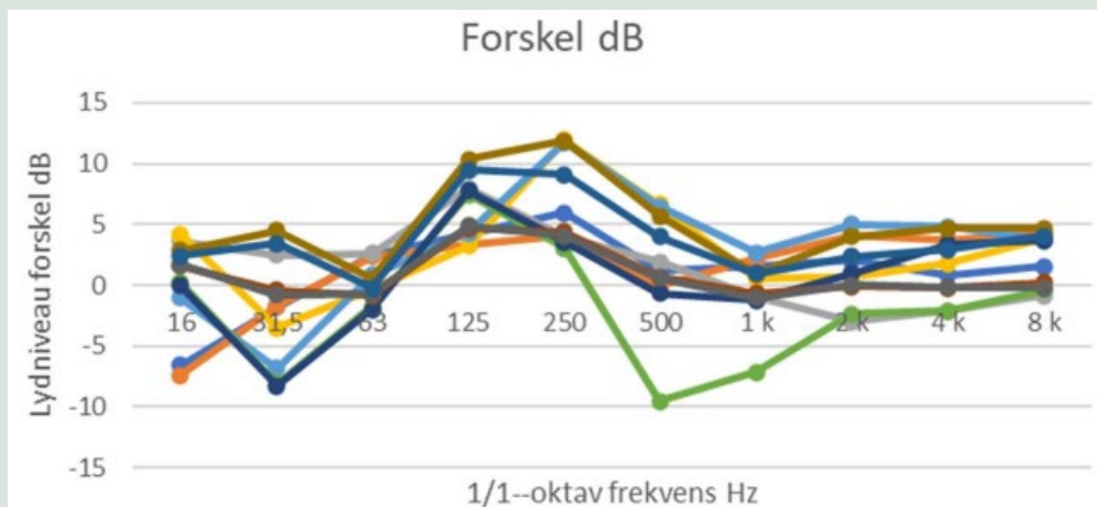
FIGUR 8. Målt lyddæmpning inde i skibet.
