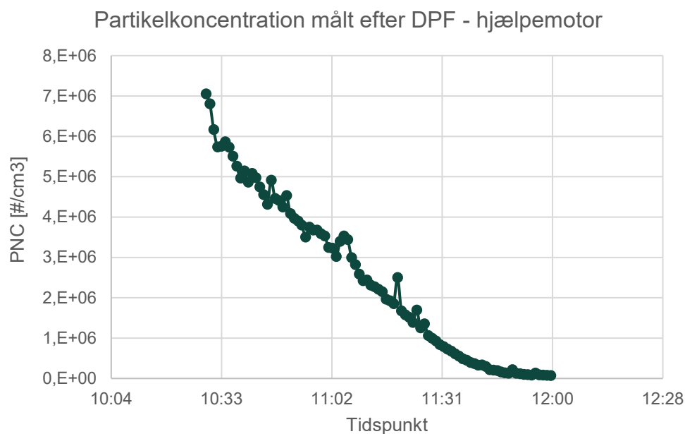
FIGUR 11. Udvikling i målt partikelkoncentration efter DPF på hjælpemotor.
