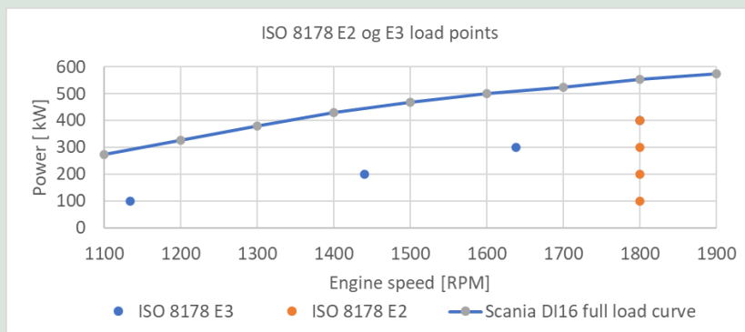
FIGUR 5. Belastningspunkter anvendt i afprøvningen.
