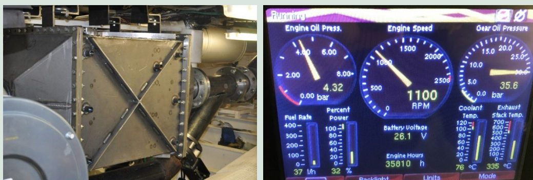
FIGUR 15. Billede af filterkassen på Hundested-Rørvig-færgen med udtag til de forskellige måle-udtag (t.v.) og billede af display hvor motorens omdrejningstal løbende blev aflæst og noteret fra motorens informationsskærm (t.h.).
