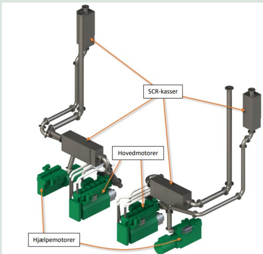
FIGUR 21. Installation af SCR på M/S Pernilles motorer.
