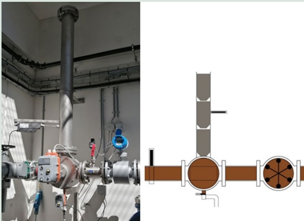
FIGUR 3. Magasin og rensegrisaftsender til bløde og coatede rensegrise, udviklet af Svendborg Motorværksted ApS.
