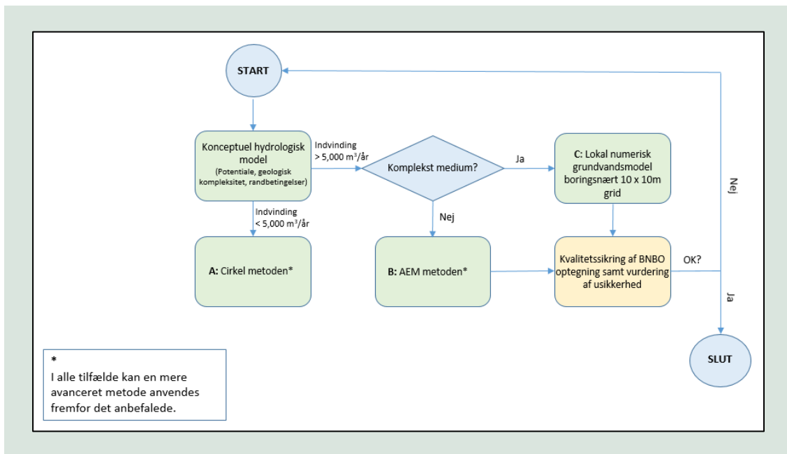
FIGUR 3. Flowdiagram, der skal anvendes til valg af BNBO beregningsmetode.
