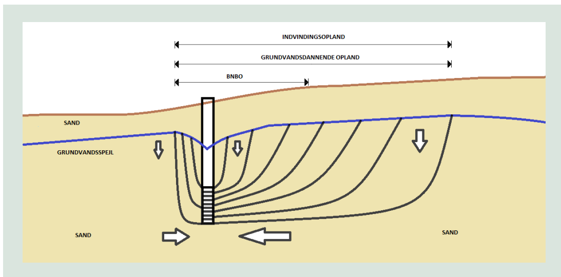
FIGUR 1. Illustration af et BNBO i et frit sandmagasin uden dæklag.
