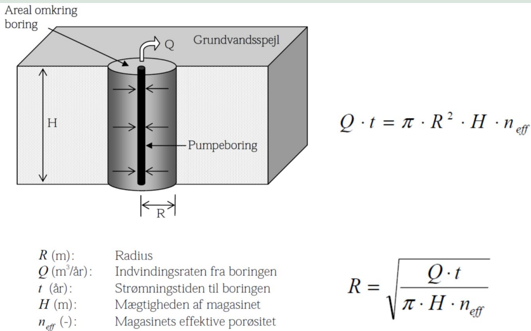
FIGUR 4. Cirkelmetoden til beregning af BNBO.
