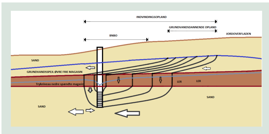
FIGUR 2. Illustration af et BNBO for en boring i et spændt sandmagasin, overlejret af et lerdæklag og et øvre frit sand magasin.
