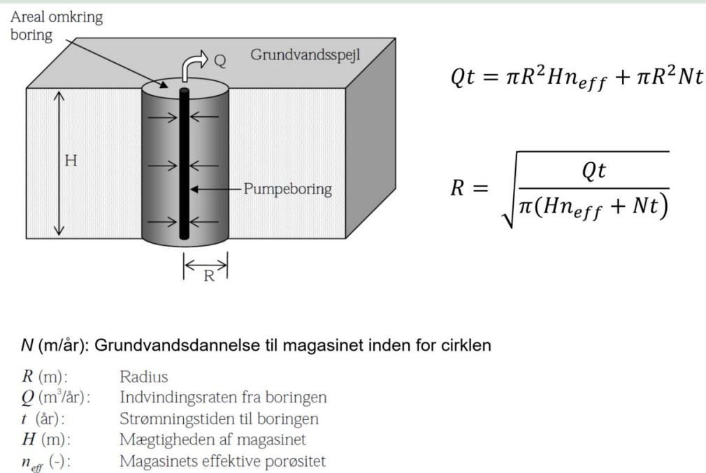
FIGUR 5. Cirkelmetoden til beregning af BNBO med grundvandsdannelse til magasinet.
