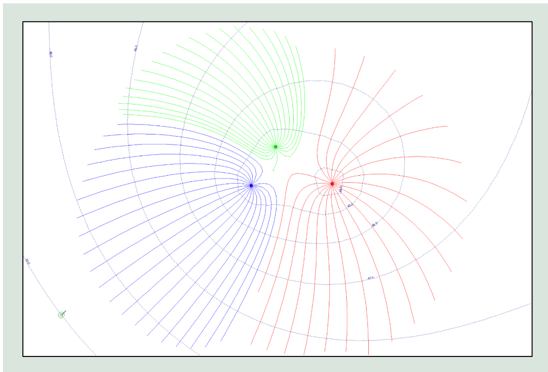
FIGUR 7. Eksempel på BNBO beregnet med en AEM-model med 3 indvindingsboringer.
