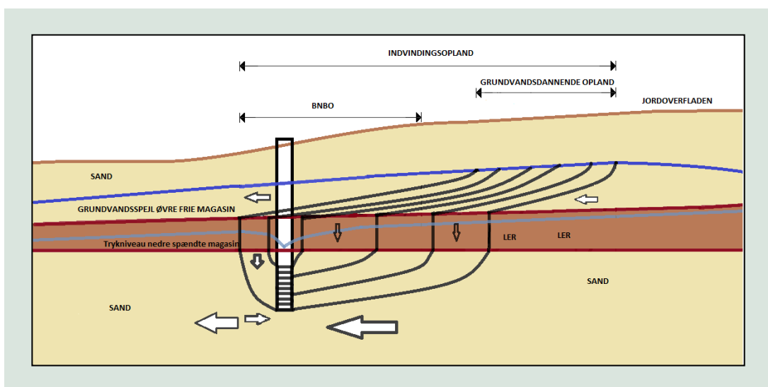
FIGUR 6. Illustration af et BNBO for en boring i et spændt sandmagasin, overlejret af et ler-dæklag og et øvre frit sand magasin 9 .
