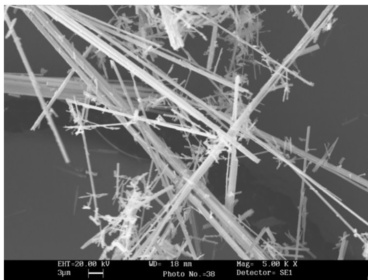
Figur 1: SEM-billede af asbestfibre taget ved en forstørrelse på 5.000 gange.
