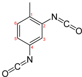
FIGURE 3 2,4-TDI.
