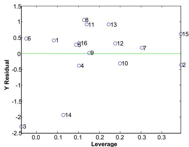
FIGUR 8 PRØVERNES INDFLYDELSE (LEVERAGE) PÅ KORRELATIONEN MOD FEJLEN I KORRELATIONSEVNEN VED PRÆDIKTION AF PRØVENS VÆRDI (Y RESIDUAL). PLOTTET BRUGES VED UDPEGNING AF OUTLIERS I FORBINDELSE MED EN PLS KORRELATIONSANALYSE.
