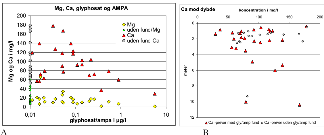
FIGUR 3.15 A - GLYPHOSAT OG AMPAKONCENTRATION MOD MG OG CAINDHOLD. DER ER ANVENDT DEN MAKSIMALE GLYPHOSAT/AMPAKONCENTRATION I DEN ENKELTE VANDPRØVE. B – CAKONCENTRATION I PRØVER MED/UDEN FUND AF GLYPHOSAT MOD PRØVEDYBDE.
