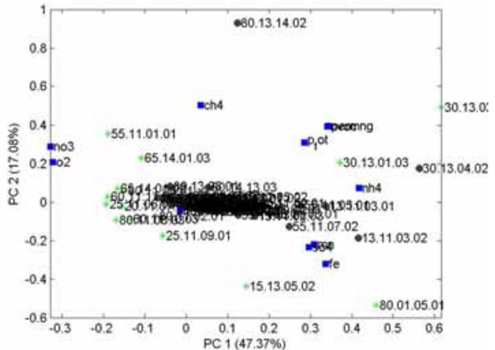
FIGUR 5 BILOT MED PROJICEREDE DATA.
