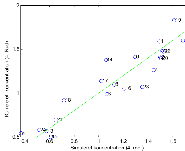
FIGUR 9 EKSEMPEL PÅ FIGUR DER VISER KORRELATIONENS PRÆDIKTIONSEVNE.
