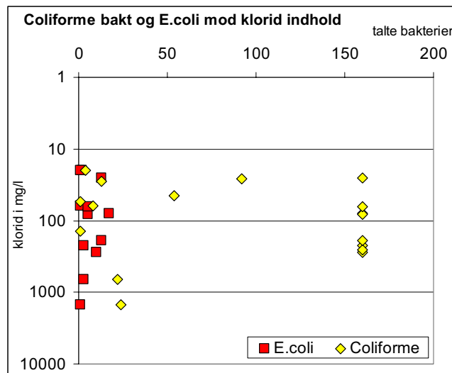
FIGUR 3.11 COLIFORME BAKTERIER OG E.COLI MOD KLORIDINDHOLD I HÅNDBORINGER. HYPOTESE: ET LAVT KLORIDINDHOLD VIL VISE INFILTRATION AF REGNVAND -> MEDDRIVNING AF BAKTERIER FRA OVERFLADE. MAKSIMUMSGRÆNSEN FOR TALLE BAKTERIER ER 160 100/ML.
