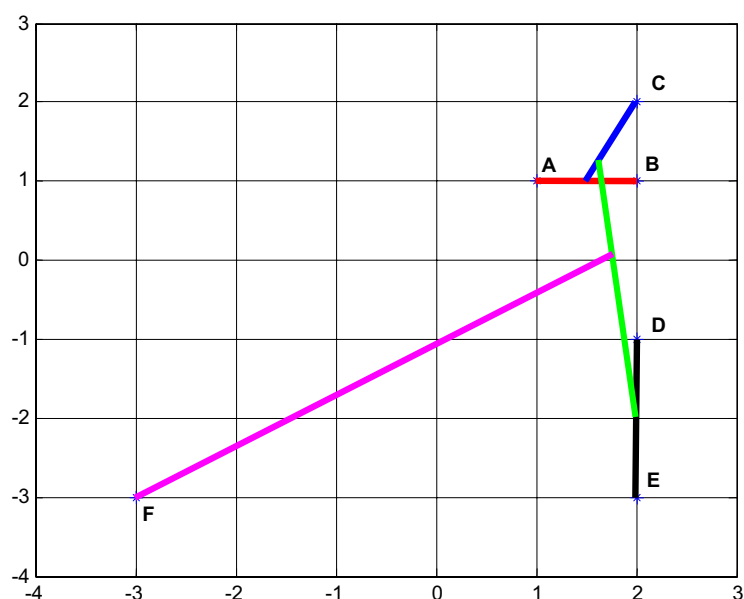
FIGUR 6 XY PLOT DER VISER AFSTANDBEREGNING FOR DATASÆTTET I TABEL 1. DE ENKELTE PRØVERS EGENSKABER ER ANGIVET VED GRIDNETTETS KRYDSPUNKTER. DE FARVEDE LINIER FORBINDER DE PRØVER ELLER BEREGNEDE GENNEMSNITSPOSITIONER AF PRØVERNES EGENSKABER SOM SUCCESSIVT GENNEM ANALYSEN LIGGER HINANDEN NÆRMEST, STARTENDE MED DEN RØDE LINIE OG AFSLUTTENDE MED DEN LILLA.
