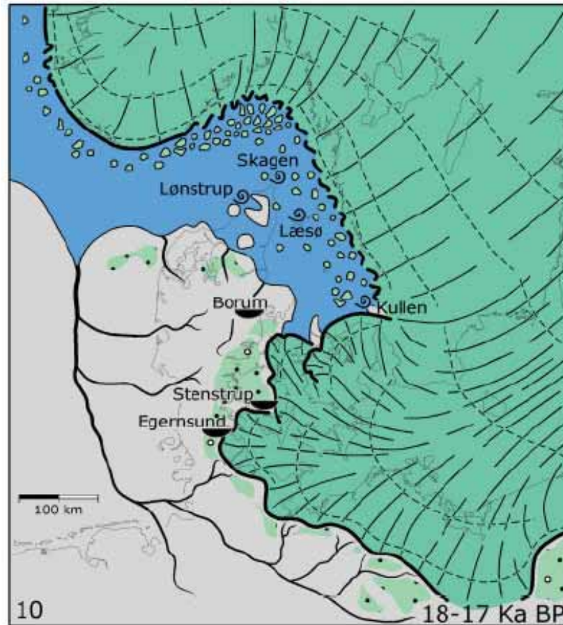
FIGUR 1.1 PALEOGEOGRAFISK REKONSTRUKTION FOR DEN UNGBALTISKE IS' UDBREDELSE I PERIODEN 18.000- 17.000 ÅR BP. DEN MAKSIMALE UDBREDELSE DÆKKED I PERIODEN 19.000-18.000 ÅR BP DELE AF ØSTJYLLAND, FRA HOUMARK-NIELSEN & KJÆR, 2003.
