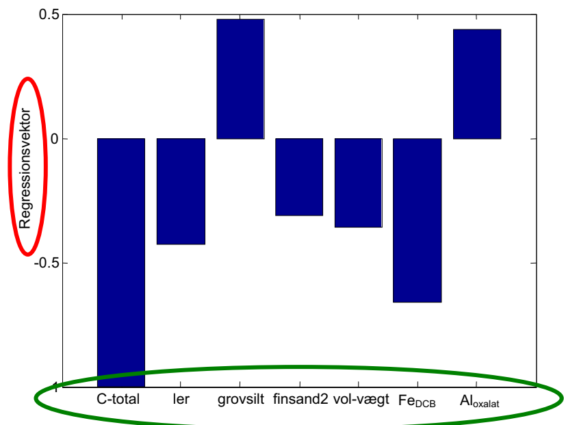
FIGUR 10 EKSEMPEL PÅ FIGUR DER VISER DE UAFHÆNGIGE VARIABLES INDFLYDELSE PÅ KORRELATIONENS EVNE TIL PRÆDIKTION AF DE AFHÆNGIGE VARIABLE. DE TILFØJEDE FREMHÆVELSER ER FORKLARET YDERLIGERE I TEKSTEN HERUNDER.
