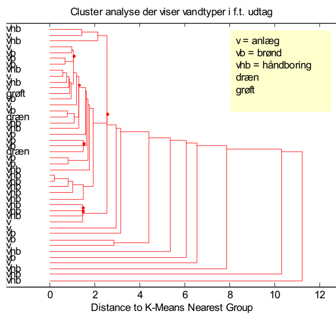
FIGUR 3.17 VANDTYPER FRA FORSKELLIGE UDTAG I FORHOLD TIL HOVEDBESTANDDELE, AMPA OG BAM.
