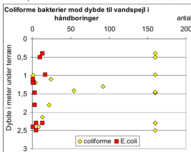
FIGUR 3.10 HÅNDBORINGER – FUND AF COLIFORME BAKTERIER OG E.COLI MOD DYBDE TIL VANDSPEJLET I HÅNDBORINGER. MAKSIMUMSGRÆNSEN FOR TALLEDE BAKTERIE ER 160/100ML.
