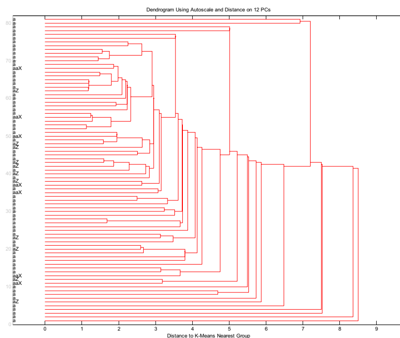
FIGUR 14 TEST AF PRØVER FRA BRØNDE FRA STORSTRØMS AMT MED ALLE INTERVIEW DATA OG UORGANISKE PARAMETRE.
