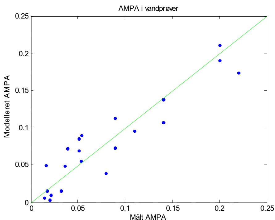
FIGUR 23 PLS MODELLENS PRÆDIKTIONSEVNE. DER ER MEDTAGET BRØNDE, ANLÆG OG HÅNDBORINGER MED FUND SAMT KEMIDATA OG ANDRE INDSAMLEDE DATA.
