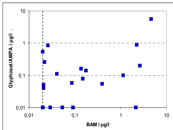
FIGUR 3.4 MÅLTE MAKSIMUMKONCENTRATIONER FOR BAM, GLYPHOSAT/AMPA I VANDPRØVER UDTAGER I ELLER VED 28 ANLÆG – DER ER MEDTAGET DEN STØRST MÅLTE KONCENTRATION FOR HVERT ANLÆG FOR BAM OG FOR GLYPHOSAT/AMPA. DETEKTIONSGRÆNSEN ER 0,02 FOR BAM MENS DEN ER 0,01 FOR GLYPHOSAT/AMPA. DEN STIPLEDE LINIE VISER DETEKTIONSGRÆNSEN FOR BAM.
