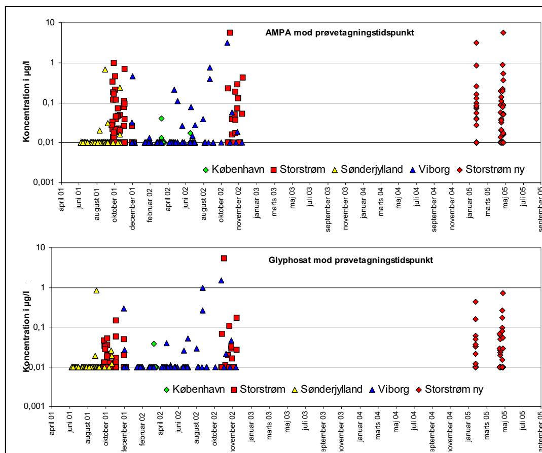
FIGUR 3.6 FUND AF GLYPHOSAT OG AMPA FRA DEN TIDLIGERE UNDERSØGELSE I 4 AMTER OG FRA DENNE UNDERSØGELSE. ALLE ANALYSER ER VIST MOD PRØVETAGNINGSTIDSPUNKT. DETEKTIONSGRÆNSEN ER PÅ 0,01 µG/L OG DEN ALTOVERVEJENDE DEL AF VÆRDIERNE PÅ 0,01 µG/L ER MÅLINGER UNDER DETEKTIONSGRÆNSEN. STORSTRØM NY – ANALYSER FRA ANLÆG SOM BLEV BESØGT I 2005.
