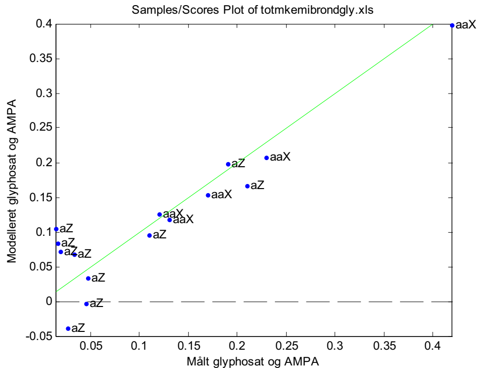
FIGUR 21 PLS MODELLENS PRÆDIKTIONSEVNE. DER ER MEDTAGET BRØNDE MED FUND SAMT KEMIDATA OG INTERVIEW DATA.
