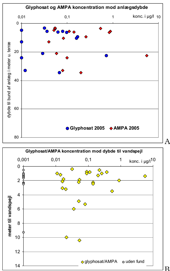
FIGUR 3.2 A - GLYPHOSAT OG AMPA KONCENTRATIONER MOD ANLÆGGENES DYBDE MÅLT I METER FRA TERRÆN TIL ANLÆGGENES BUND (BUND AF GRAVET BRØND ELLER BUND AF BØRING). DER ER KUN MEDTAGET ANALYSER GJENNEMFØRT I 2005. B - GLYPHOSAT/AMPA MAKSIMUMKONCENTRATION I VANDPRØVER MOD PRØVETAGNINGSDYBDEN / GRANDVANDSPEJLETS BELIGGENHED I HÅNDBØRINGER OG BRØNDE.
