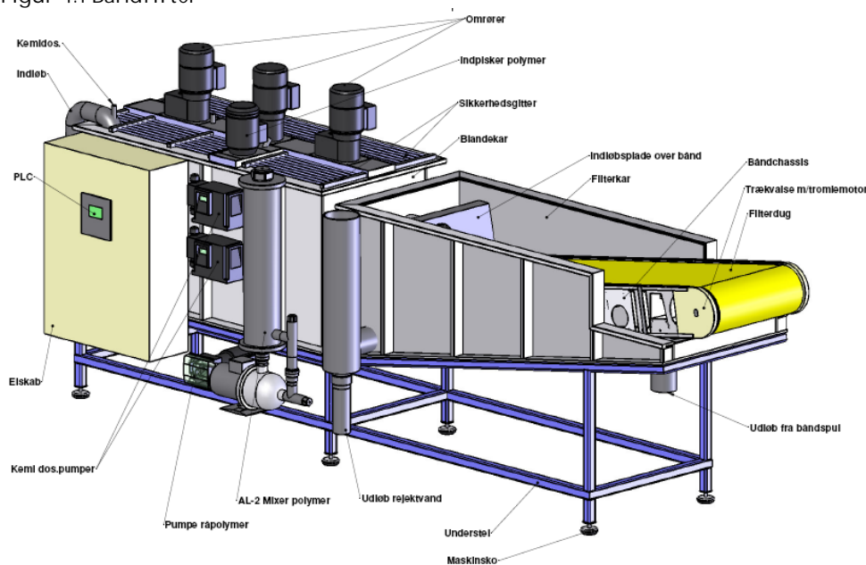
Figur 4.1 Båndfilter
